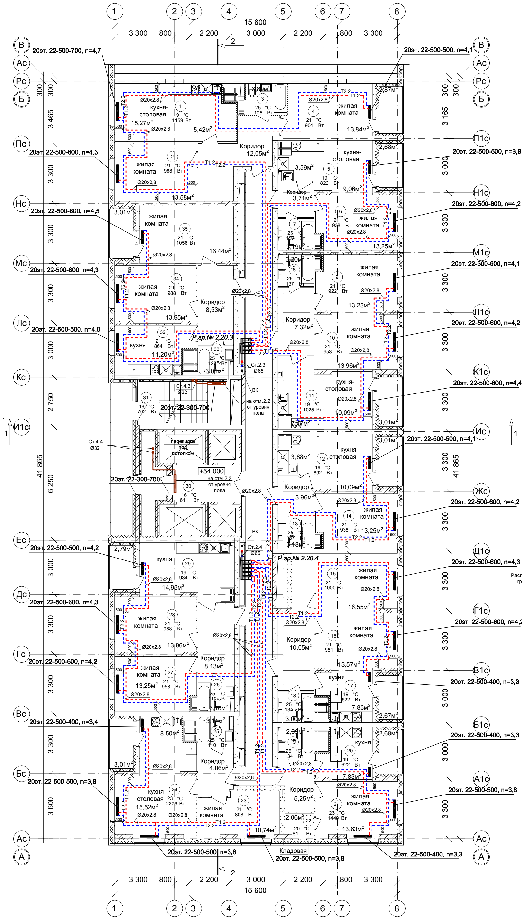
Компоновочная схема
