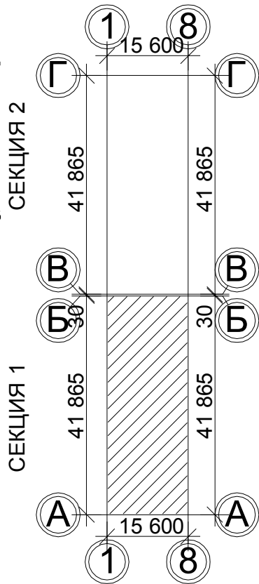
Компоновочная схема
